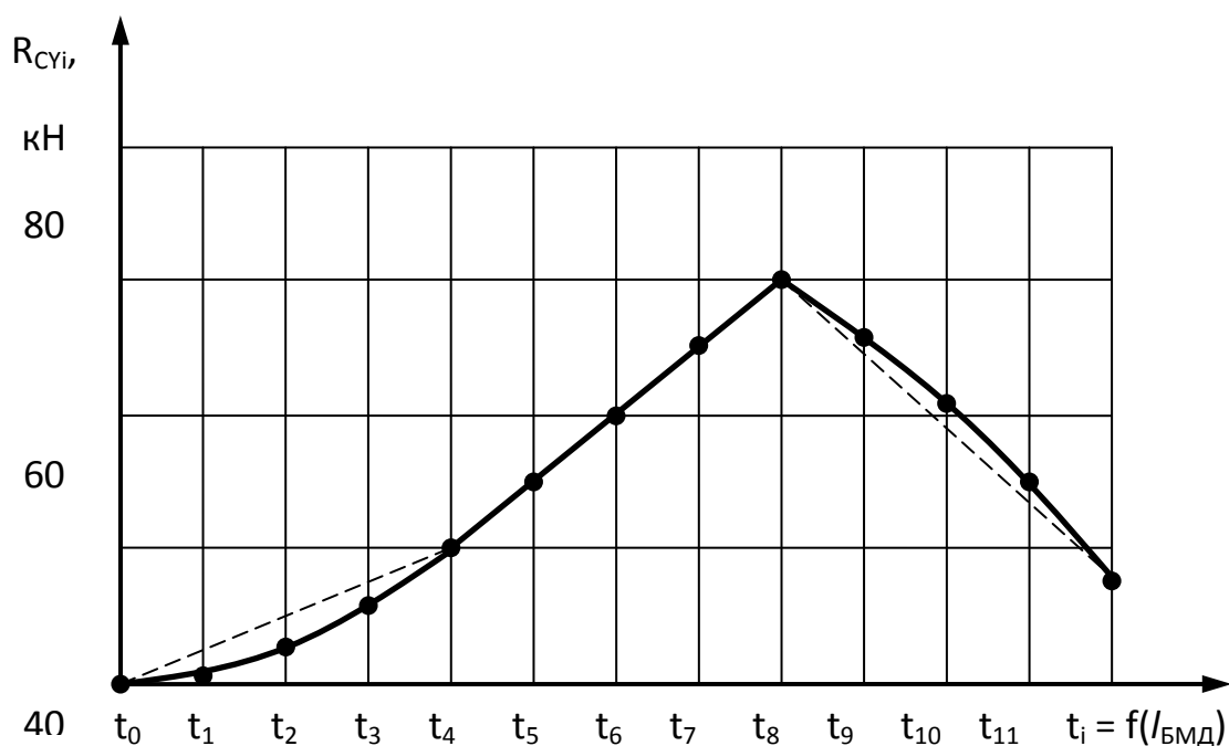
Рисунок 6 – Изменение нагрузки на опору С в направлении оси 0Y.
