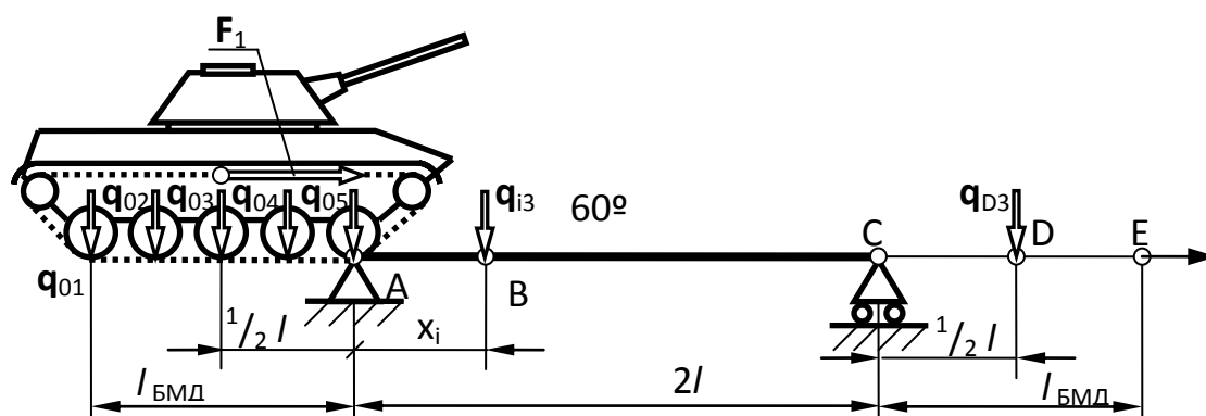
Рисунок 1 – Нагружение колейного моста БМД, перемещающейся с постоянной скоростью в линейном масштабе 1 : 10 (весовом 1 : 1 000).
