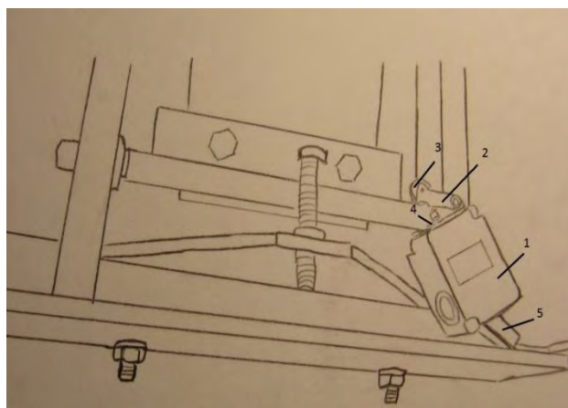
Рисунок 3 – Блок управления устройством для активации качающейся мишени «Свингер»: 1 – корпус; 2 – замыкатель контакта; 3 – ролик; 4 – пластина; 5 – разъем для подключения внешнего устройства
