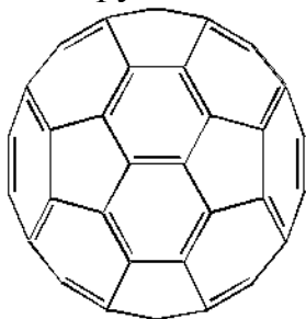
Модель молекулы фуллерена C 60 .
